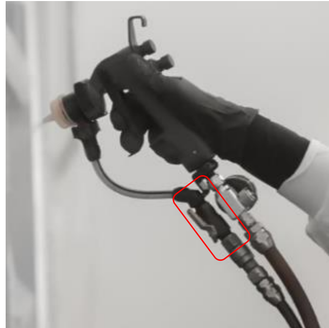
Ejemplo de una válvula de bola montada en una pistola de pulverización
